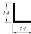
AL-31 0.171 kg/m
