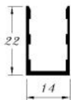
AL-67 0.170 kg/m
