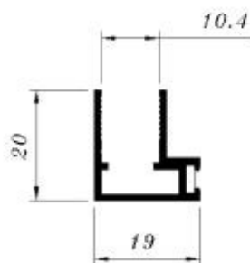
AL-14 0.263 kg/m
